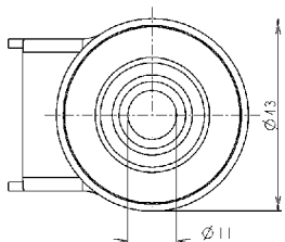
Upevnenie na stredový otvor Ø 11 na otočné vidlice série 252
