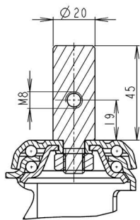
upínanie na hladký čap Ø 20x45 s pričným otvorom označenie - 373.....H1
