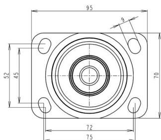
Upevňovacia príruha štvorhranná-typ P33 na otočné vidlice série 323, 383
