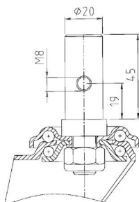
Upínanie na hladký čap Ø 20x45 s priečnym otvorom označenie - 372.....H1
