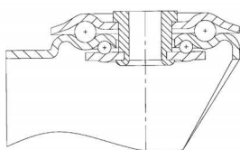
Otočná vidlica typ 452
