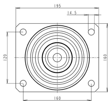
Typ P8 - na kolesá série 628,638
