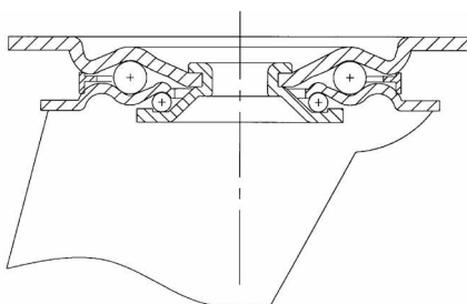
otočná vidlica typ 623
