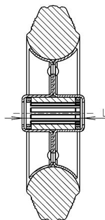
Kolesá s ihlovým ložiskom
