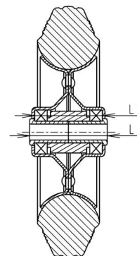
Kolesá s guľičkovým ložiskom
