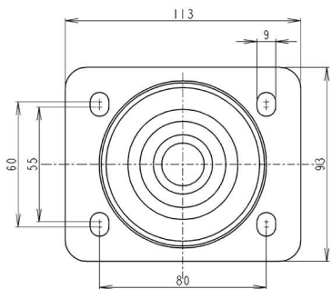
Upevňovacia príruha štvorhranná - typ P44 na kolesá série 420,420B,430
