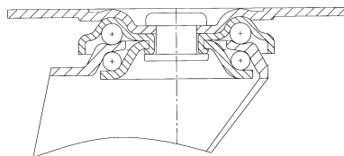
Otočná vidlica typ 322
