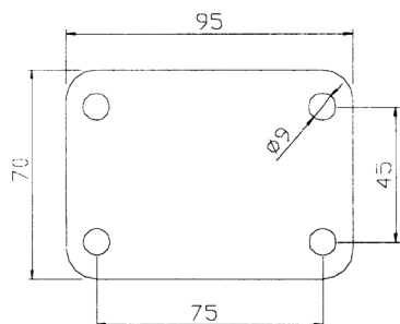
Upevňovacia príruha štvorhranná-typ P3 na vidlice série 322,332
