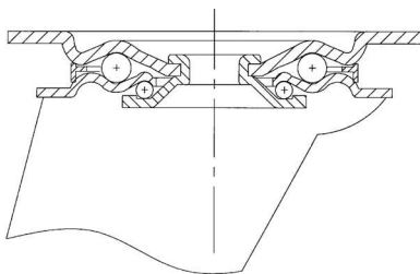
Otočná vidlica typ 620
