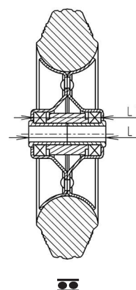
Kolesá s guľičkovým ložiskom
