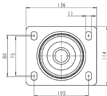
Upevňovacia príruha štvorhranná - typ P66 na kolesá série 620,620F,630
