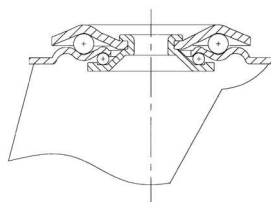
Otočná vidlica typ 653
