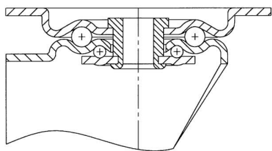
Otočná vidlica typ 420
