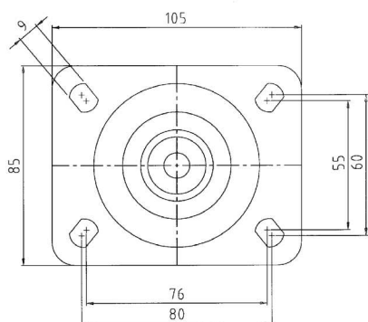
Typ P4 - na kolesá série 422,432
