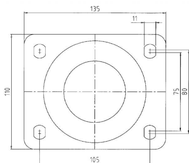
Typ P6 - na kolesá série 623,633
