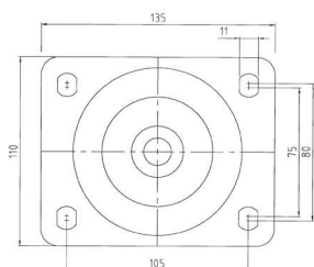
Upevňovacia príruha štvorhranná-typ P6 na vidlice série 624,634
