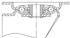
Otočná vidlica typ 423
