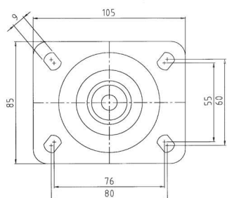
Upevňovacia príruha štvorhranná-typ P4 na kolesá série 422,422B,432
