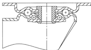
Otočná vidlica typ 422
