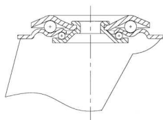
Otočná vidlica typ 653
