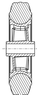
Kolesá s klzným uložením
