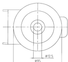
Upevnenie na stredový otvor \varnothing 12,5 na otočné vidlice série 653
