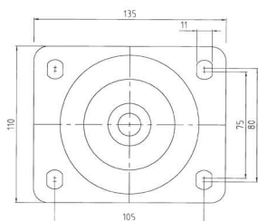
Upevňovacia príruha štvorhranná-typ P6 na kolesá série 623,623F,623T,633
