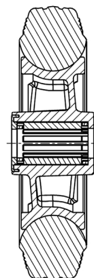
Kolesá s ihlovým ložiskom
