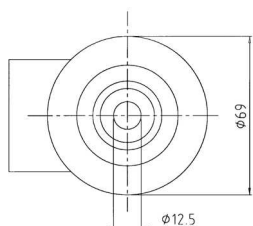
Upevnenie na stredový otvor \varnothing 12,5 na otočné vidlice série 452
