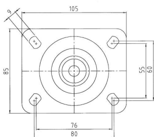
Upevňovacia príruha štvorhranná-typ P4 na kolesá série 423,433
