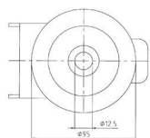
Upevnenie na stredový otvor Ø 12,5 na otočné vidlice série 653
