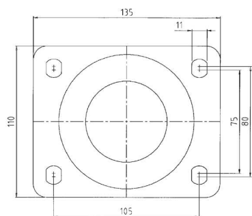
Upevňovacia príruha štvorhranná-typ P6 na kolesá série 824,834,825,834
