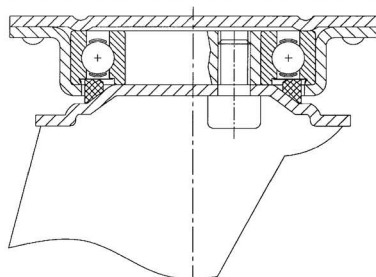
Otočná vidlica typ 824,825
