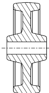
Kolesá s klzným uložením
