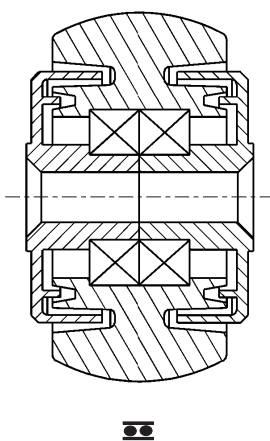
Kolesá s guľičkovými ložiskami
