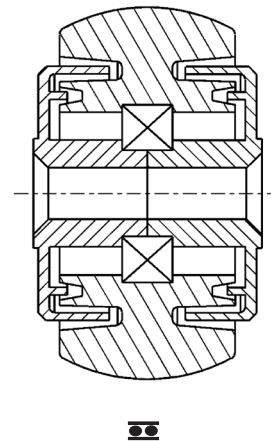
Kolesá s guľičkovým ložiskom
