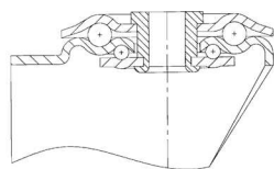
Otočná vidlica typ 453
