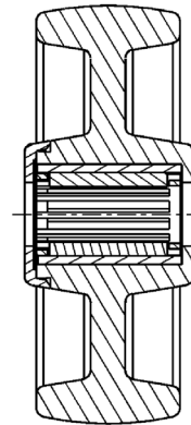
Kolesá s ihlovým ložiskom
