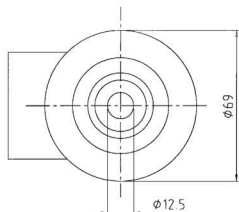
Upevnenie na stredový otvor \varnothing 12,5 na otočné vidlice série 453
