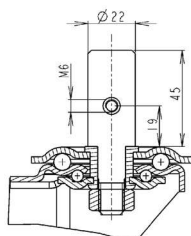
Upínanie na hladký čap \varnothing 22x45 s priečnym otvorom označenie: 473.....H1
