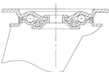
Otočná vidlica typ 824,825
