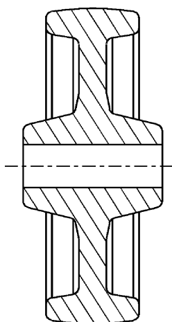
Kolesá s klzným uložením
