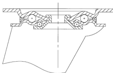
Otočná vidlica typ 623,624
