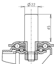
Upevnenie na hladký čap \varnothing 22x45
