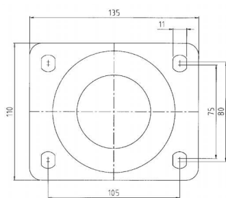
Upevňovacia príruha štvorhranná - typ P6 na kolesá série 623,624,633,634
