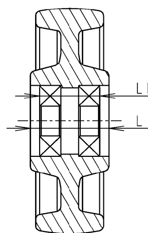
Kolesá s guľičkovým ložiskom
