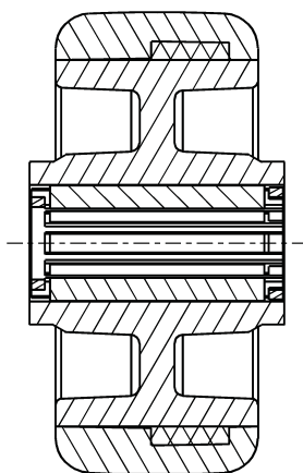
Kolesá s ihľovým ložiskom
