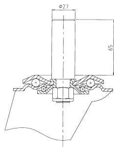
Upínanie na hladký čap Ø 27x65
