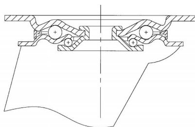
Otočná vidlica typ 624
