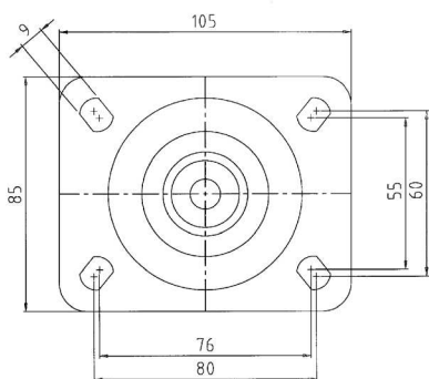
Upevňovacia príruha štvorhraná - typ P4 na kolesá série 422, 423
