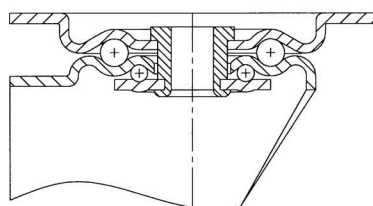
Otočná vidlica typ 422
