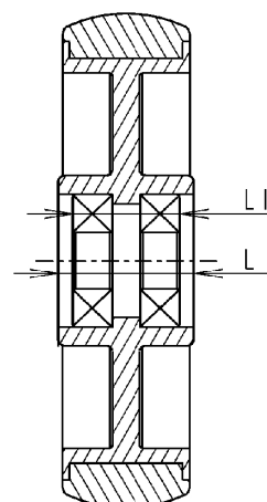
Kolesá s guľičkovým ložiskom
