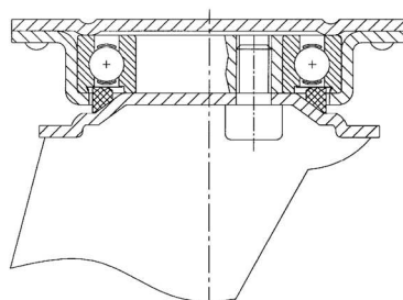
Otočná vidlica typ 824
