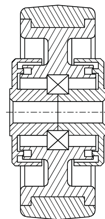
Kolesá s guľičkovým ložiskom
