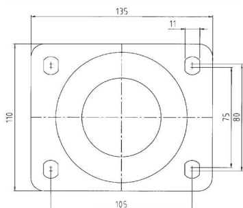
Upevňovacia príruha štvorhranná - typ P6 na kolesá série 624,634
