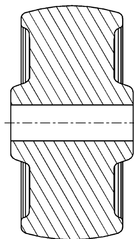
Kolesá s klzným uložením
