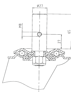
Upínanie na hladký čap Ø 27x65 s pričným otvorom označenie: 673, 674.....H1
