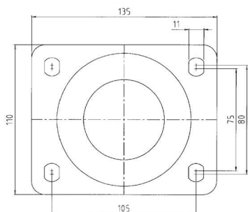
Upevňovacia príruha štvorhranná - typ P6 na kolesá série 824,834
